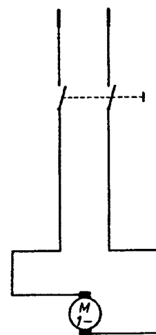
WIRING-DIAGRAM SCHALTPLAN
