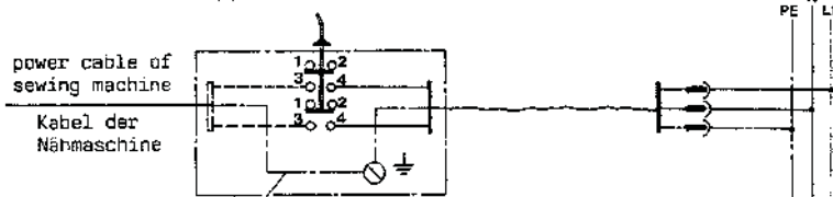
Wiring Diagram Anschlußschema
